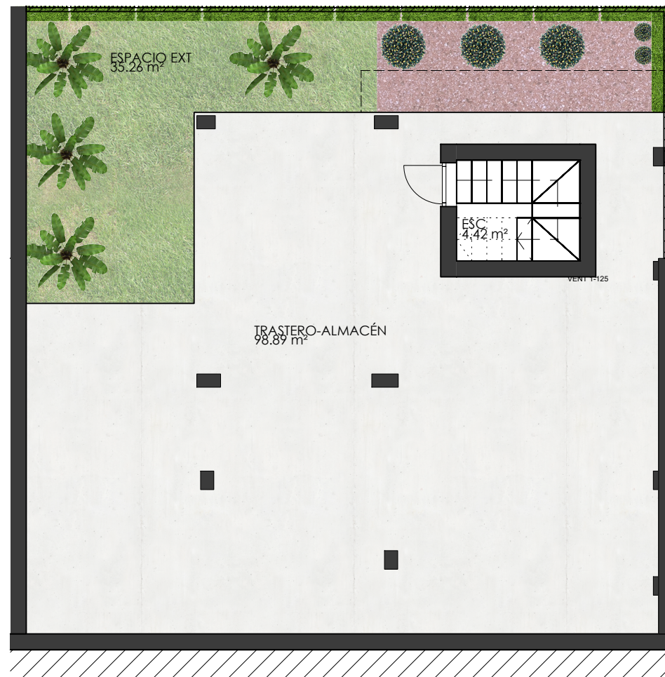
Planta Sótano
