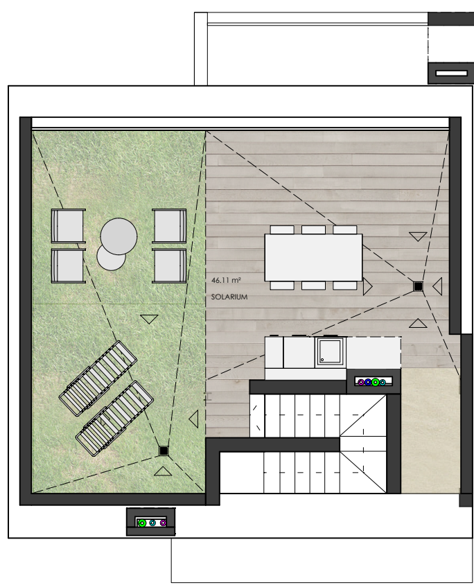
Planta Primera
