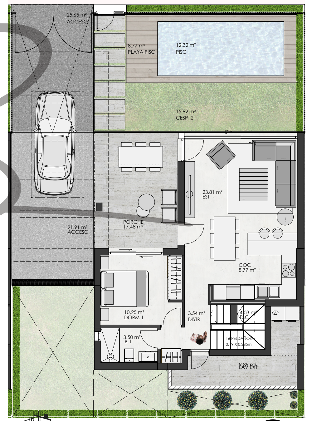
Planta Baja
