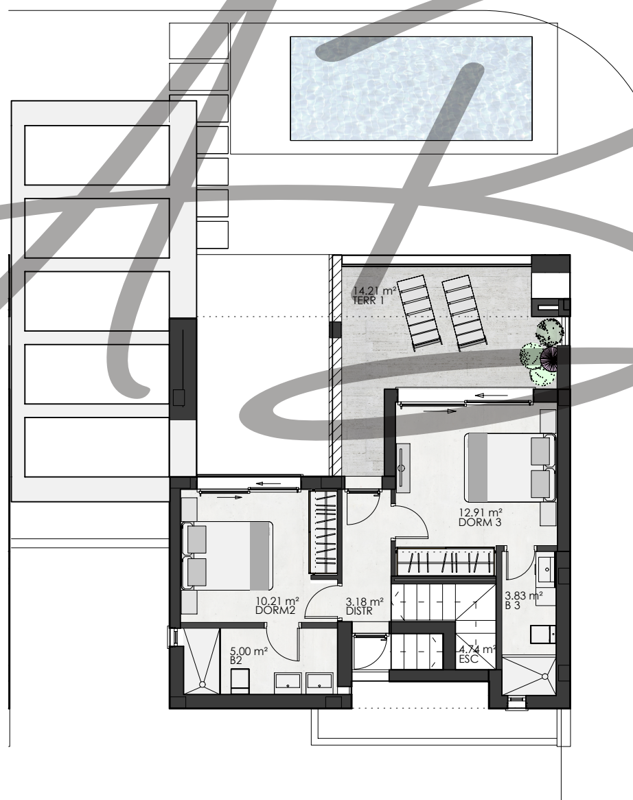
Planta Primera
