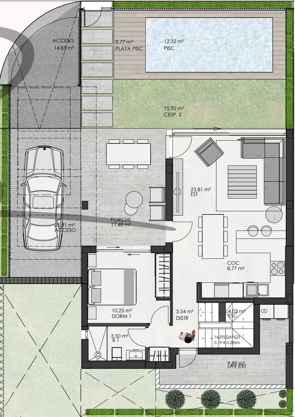
Planta Baja
